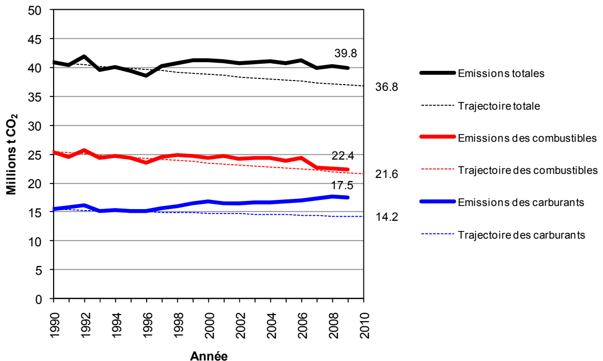
Graphique 2: Evolution des émissions de CO 2 selon la loi sur le CO 2 (1990 à 2010), en millions de tonnes de CO 2 . Les lignes en pointillé indiquent la trajectoire des émissions sans tenir compte des certificats étrangers. Les valeurs d'émissions des combustibles sont corrigées par un facteur climatique.
