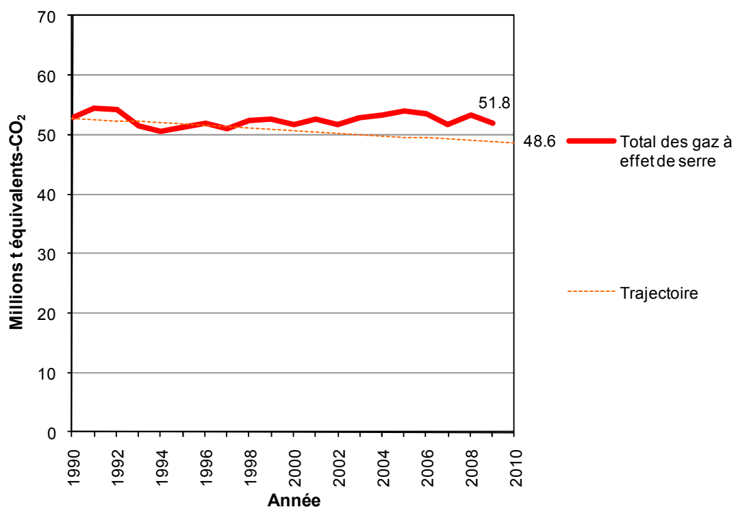
Graphique 5: Evolution des émissions de gaz à effet de serre selon le Protocole de Kyoto depuis 1990, en millions de tonnes d'équivalents-CO 2 . La ligne en pointillé marque la trajectoire que doit suivre la valeur d'émission jusqu'en 2010 (en ne tenant compte ni de l'effet de puits de carbone, ni des certificats étrangers).
