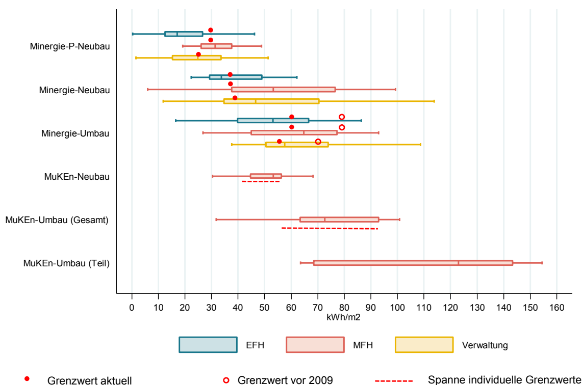
Abbildung 1: Gewichtete EKZ [kWh/m 2 ]. Die Boxen werden nur dargestellt, wenn mindestens fünf Gebäude in der jeweiligen Untergruppe vorhanden sind. Darstellung ohne Ausreisser.
