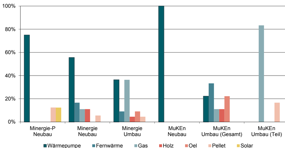
Abbildung 39: Verteilung der Hauptheizungssysteme bei den Mehrfamilienhäusern pro Standard. Bei Gebäuden mit mehreren Energieträgern wird jeweils nur der Energieträger bzw. das Heizungssystem mit dem höchsten Anteil an der Wärmeerzeugung berücksichtigt. (n=85)
