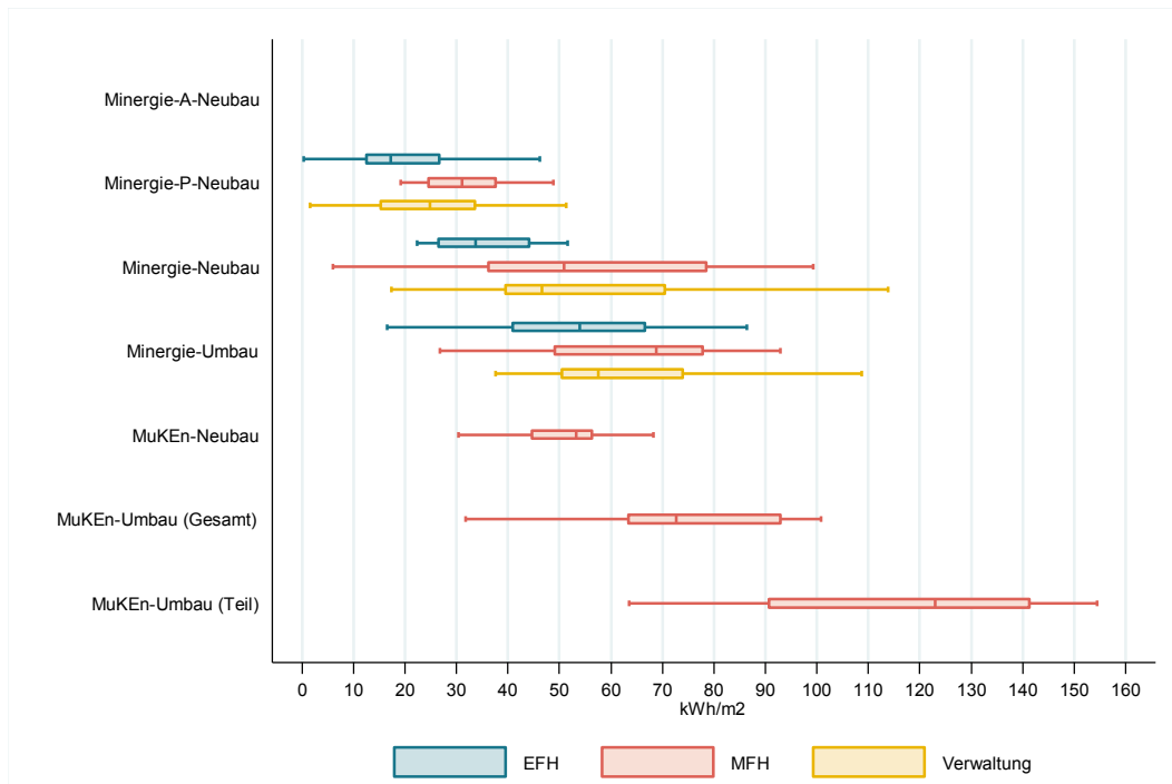
Abbildung 41: Gewichtete EKZ [kWh/m 2 ] der Gebäude mit mittlerer bis hoher Datenqualität. Die Boxen werden nur dargestellt wenn mindestens fünf Gebäude in der jeweiligen Untergruppe vorhanden sind. Darstellung ohne Ausreisser
