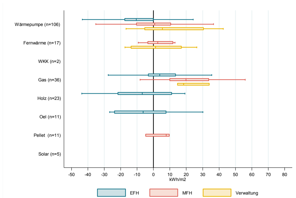
Abbildung 38: Abweichungen vom Grenzwert kWh/m 2 nach Gebäudekategorie und Hauptenergieträger. Die Boxen werden nur dargestellt, wenn mindestens fünf Gebäude in der jeweiligen Untergruppe vorhanden sind. Darstellung ohne Ausreisser. (n=212)
