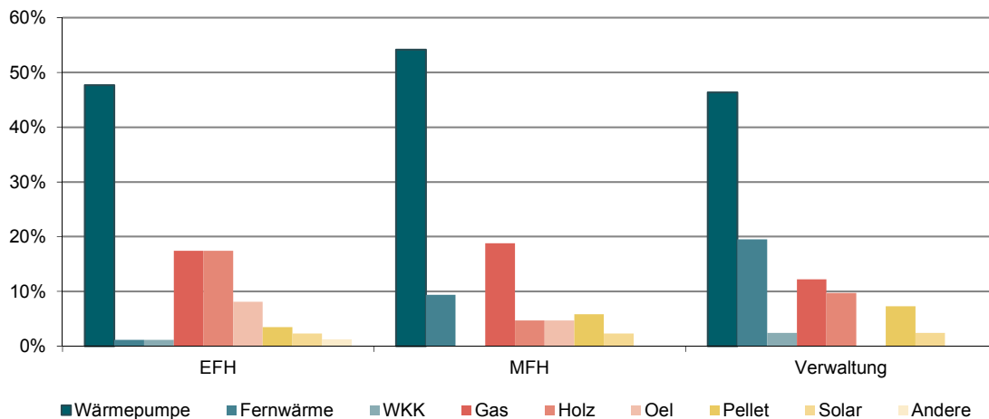
Abbildung 37: Verteilung der Hauptheizungssysteme in den drei Gebäudekategorien EFH, MFH und Verwaltung. Bei Gebäuden mit mehreren Energieträgern wird jeweils nur der Energieträger bzw. das Heizungssystem mit dem höchsten Anteil an der Wärmeerzeugung berücksichtigt. (n=213)
