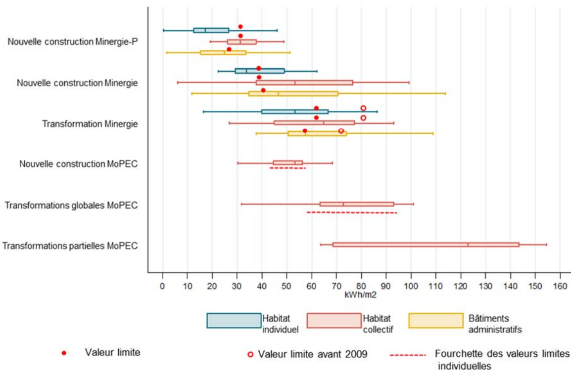
Figure 1: Indices pondérés de dépense d'énergie [kWh/m 2 ]. Les cases ne sont représentées que si le sous-groupe d'objets comporte au moins cinq bâtiments. Le graphique ne signale pas les résultats aberrants.
