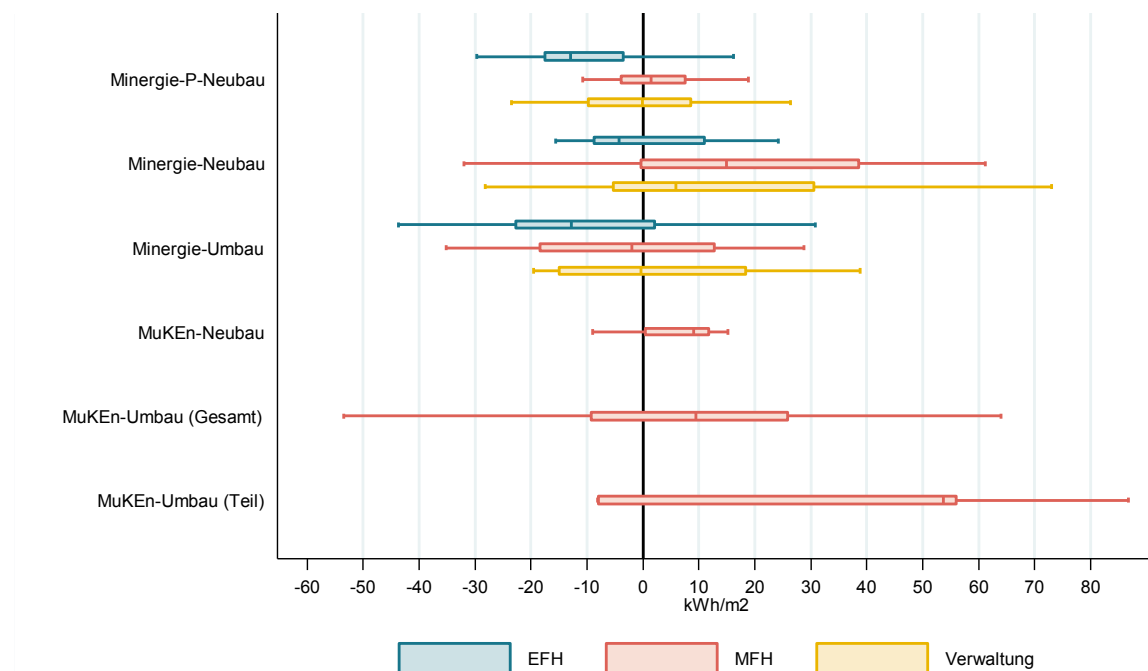
Abbildung 5: Absolute Abweichungen vom Grenzwert [kWh/m 2 ]. Die Boxen werden nur dargestellt, wenn mindestens fünf Gebäude in der jeweiligen Untergruppe vorhanden sind. Darstellung ohne Ausreisser.
