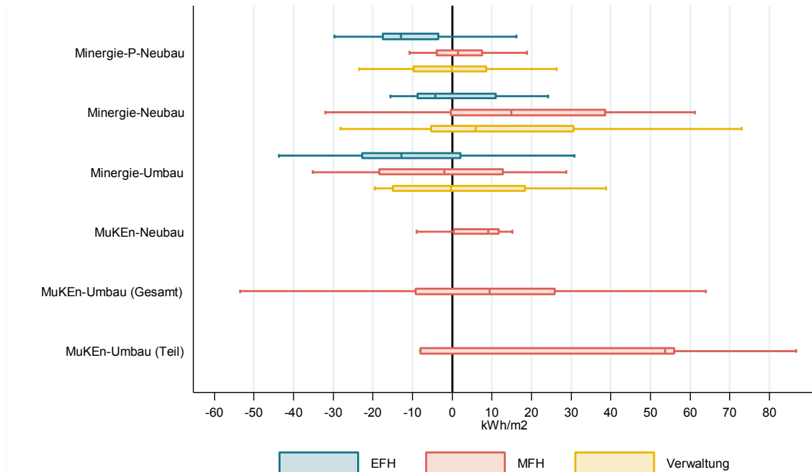
Abbildung 33: Absolute Abweichungen vom Grenzwert [kWh/m 2 ]. Die Boxen werden nur dargestellt, wenn mindestens fünf Gebäude in der jeweiligen Untergruppe vorhanden sind. Darstellung ohne Ausreisser.
