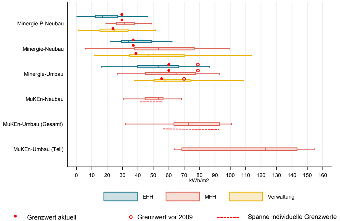
Abbildung 32: Gewichtete EKZ [ \text{kWh/m}^2 ]. Die Boxen werden nur dargestellt, wenn mindestens fünf Gebäude in der jeweiligen Untergruppe vorhanden sind. Darstellung ohne Ausreisser.
