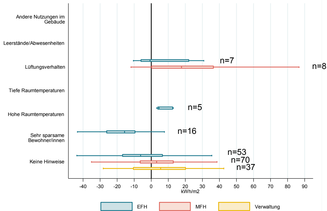
Abbildung 36: Abweichungen vom Grenzwert nach Verhaltens-Faktoren, die von den Experten/innen als möglicher Grund für ein Abweichen vom Grenzwert angegeben wurden. Die Boxen werden nur dargestellt, wenn mindestens fünf Gebäude in der jeweiligen Untergruppe vorhanden sind. Darstellung ohne Ausreisser. (n=214)
